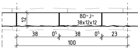
WIDOK Muru BD-J-38
