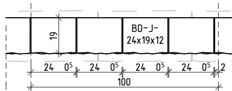
WIDOK Muru BD-J-24
